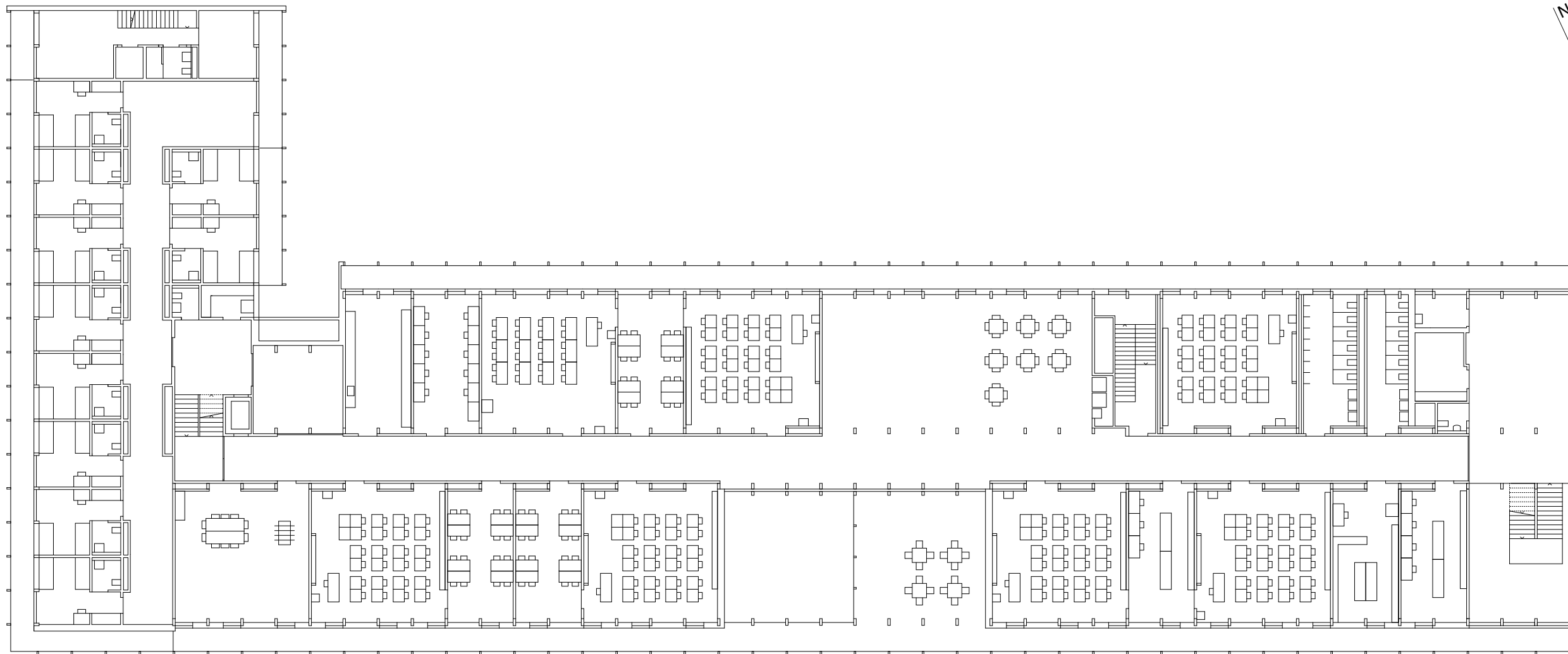
1. OBERGESCHOSS
